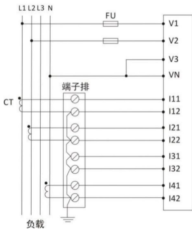
1P3W, 无PT, 2CT, I4经CT接入 系统设置: 1P3W
