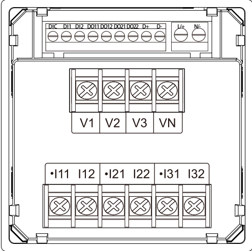
2DI+2DO 端子图
