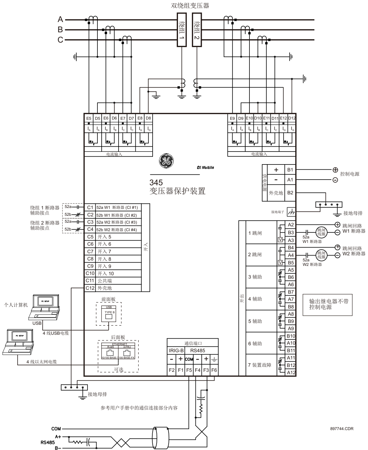
图 7: 典型接线图
