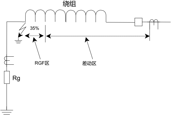
图 36:RGF 和比率差动的保护范围
