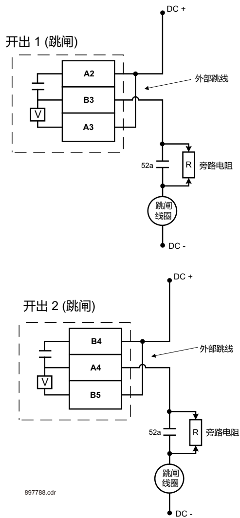
图 42: 带电压连续监视的跳闸线圈电路
