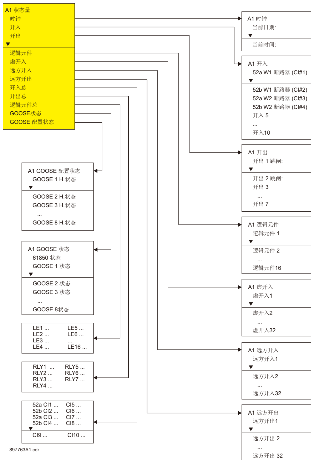
图 16: 状态菜单
