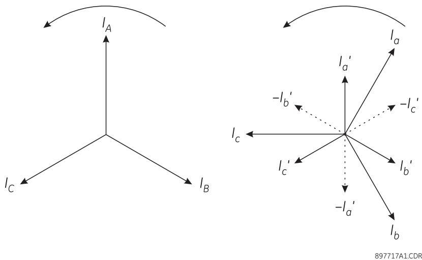
图 30: 相序 ABC 的相位图
