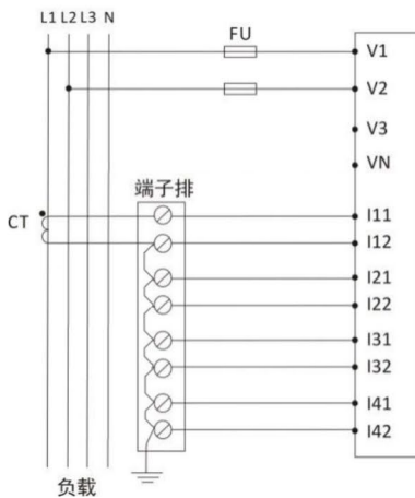
1P2W-LL, 无PT, 1CT 系统设置: 1P2W-LL
