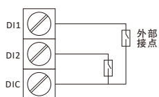
DI 接线原理图
