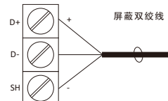
通信接线示意图
